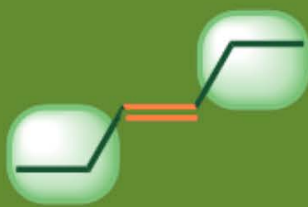
Disustituido
