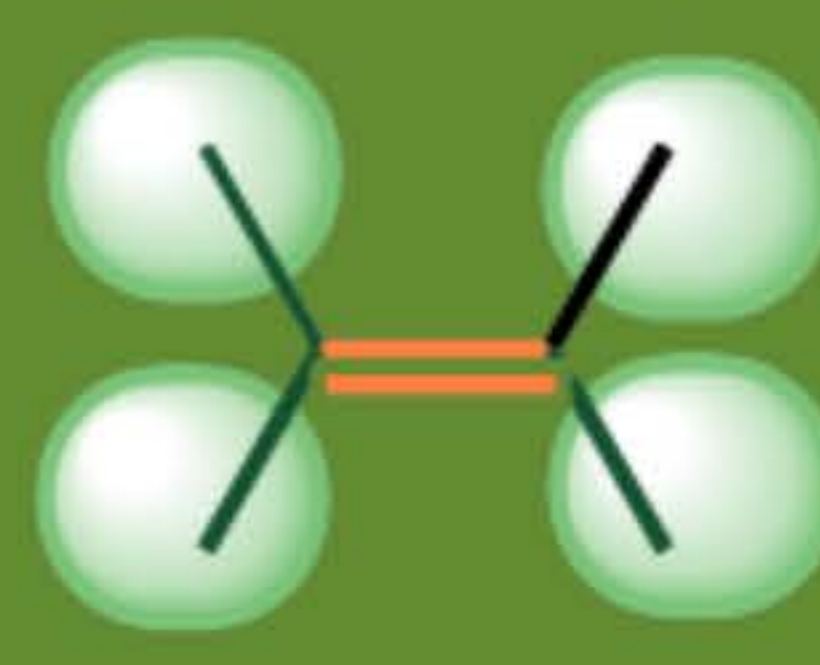
Tetrasustituido
